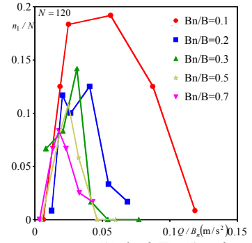
図-4 単位幅流量と遡上率
