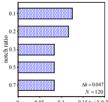
図-2 各切り欠き率における遡上率
