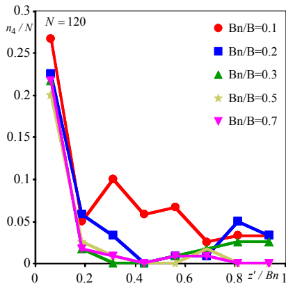
図-7 遡上位置別の遡上率
