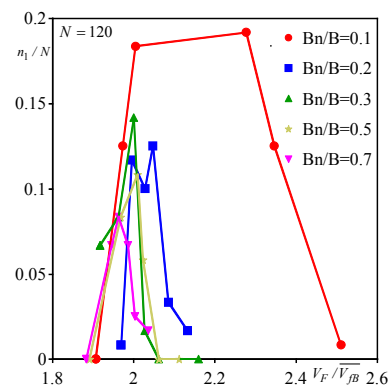
図-1 落下速度と遡上率
