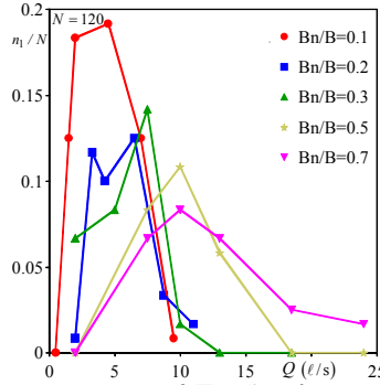
図-3 流量と遡上率
