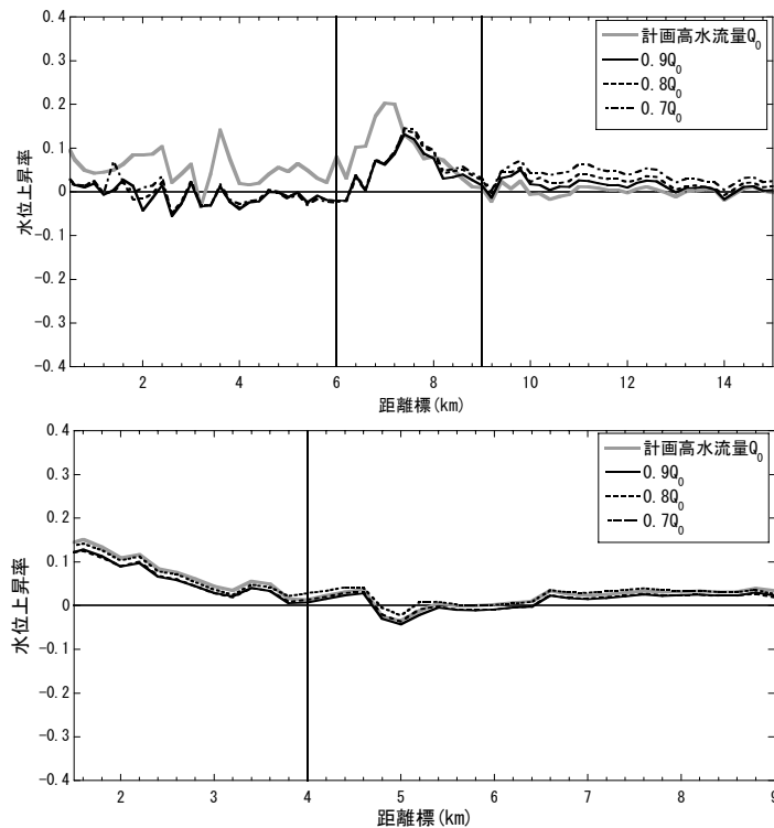
図-5 準3次元と準2次元解析の水位差と距離標との関係(上:大野川, 下:乙津川)
