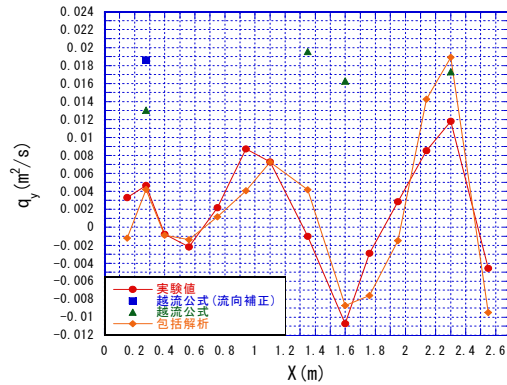
(b) 掘り込み河道(樹林帯なし, 堰あり)
