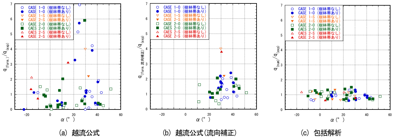
図-4 氾濫流量と流向との関係
