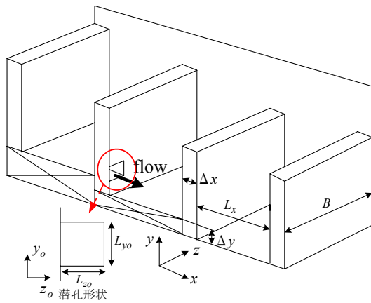
図-1 実験装置
